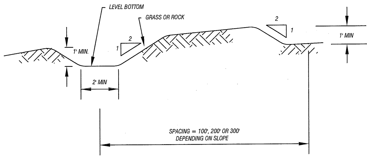
INTERCEPTOR SWALE N.T.S.
