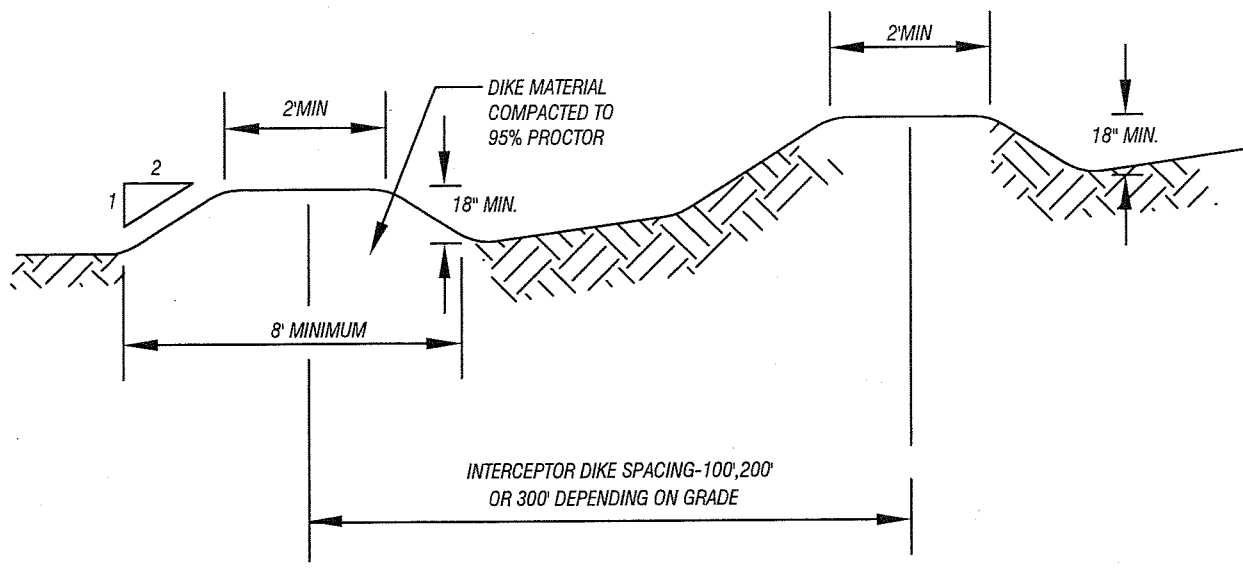
INTERCEPTOR DIKES N.T.S.
