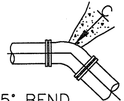
45° BEND
